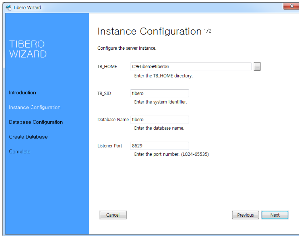
[그림 3.11] Tibero Installer - Instance Configuration (1)
