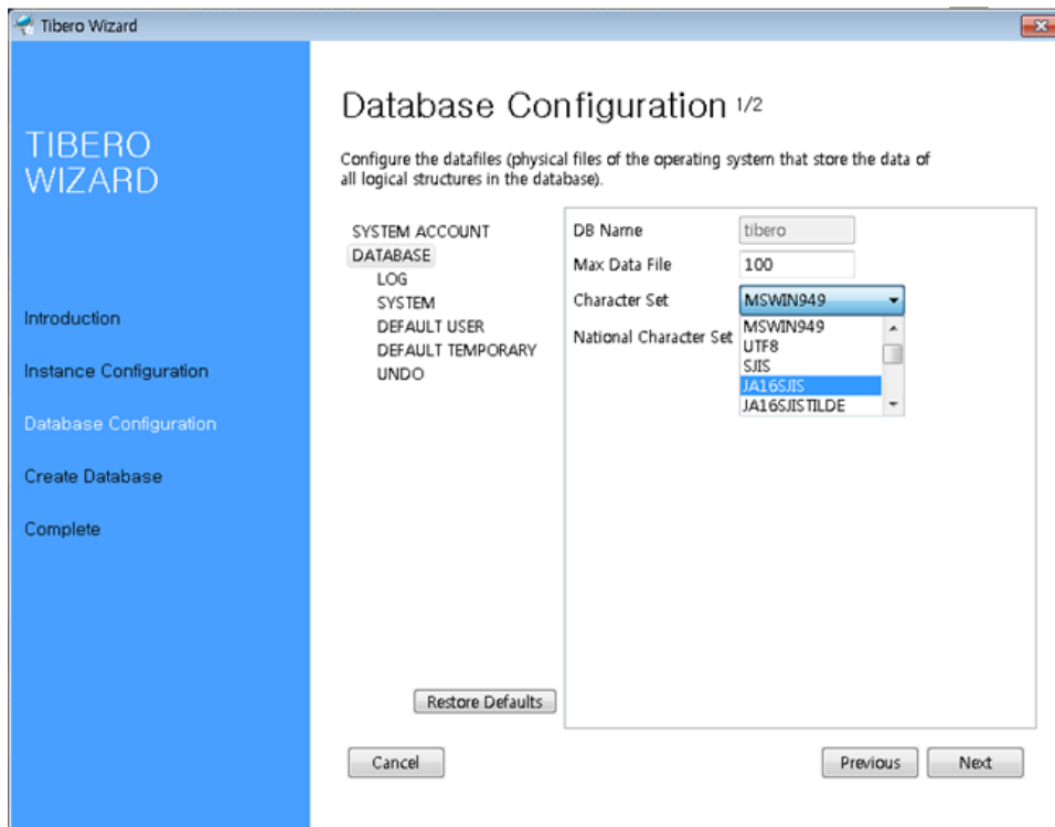
[그림 3.14] Tibero Installer - Database Configuration (2)
