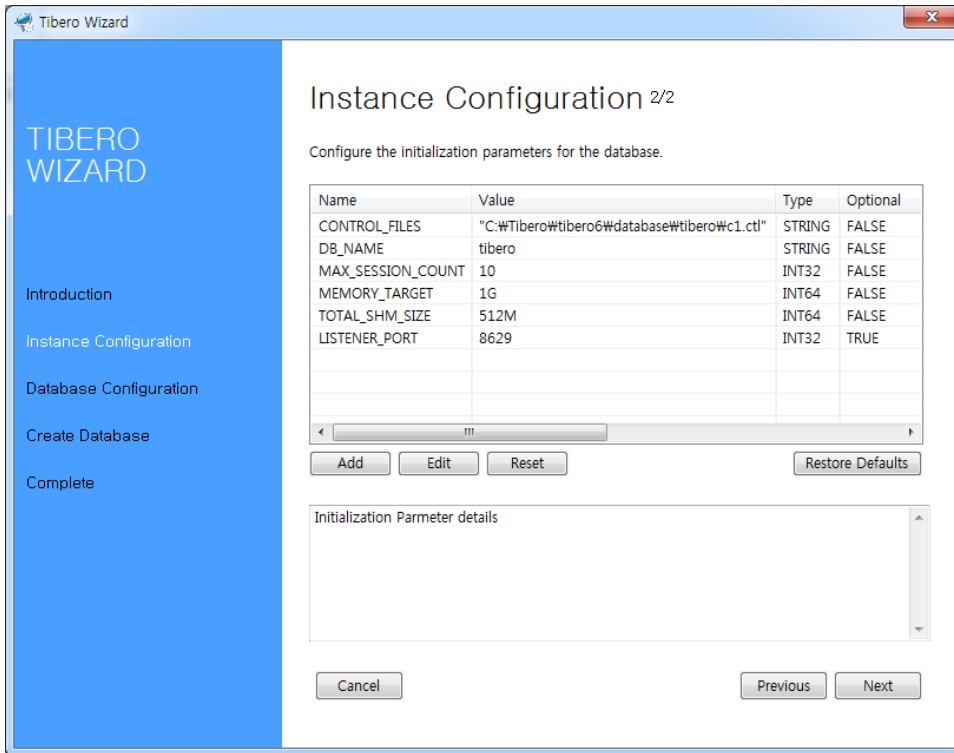
[그림 3.12] Tibero Installer - Instance Configuration (2)
